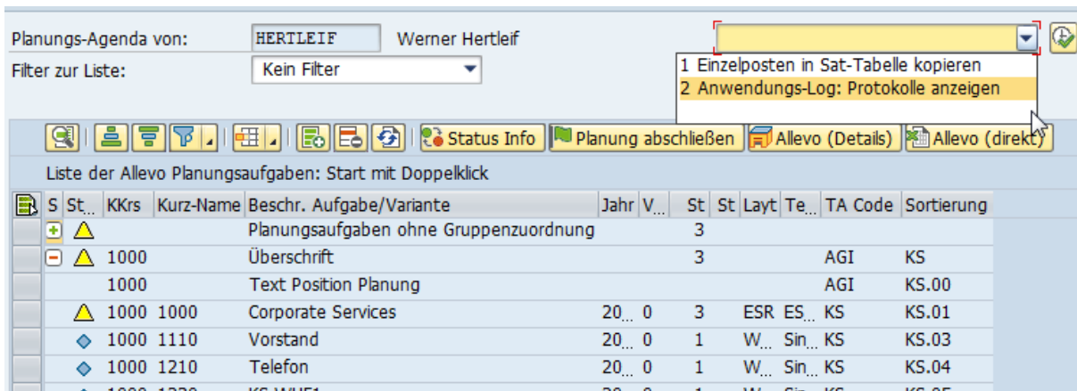
Abbildung 3-10: Zweistufige Planungs-Agenda mit Textpositionen
