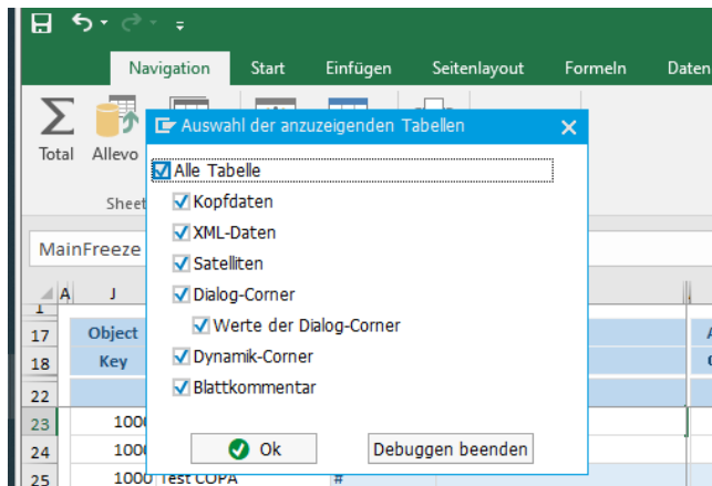
Abbildung 29-3: Auswahl der internen Tabellen (hier bei TAB2SAP)
