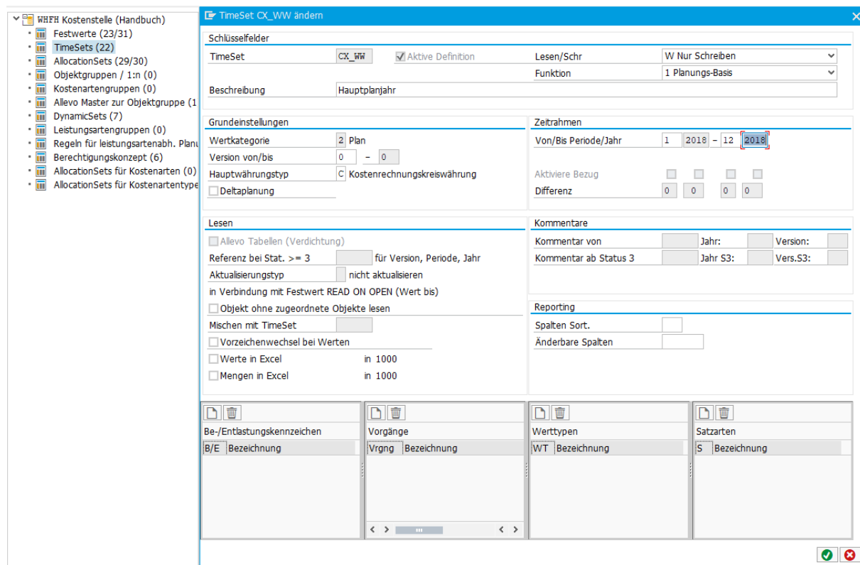
Abbildung 7-9: Merkmale zum TimeSet einrichten
