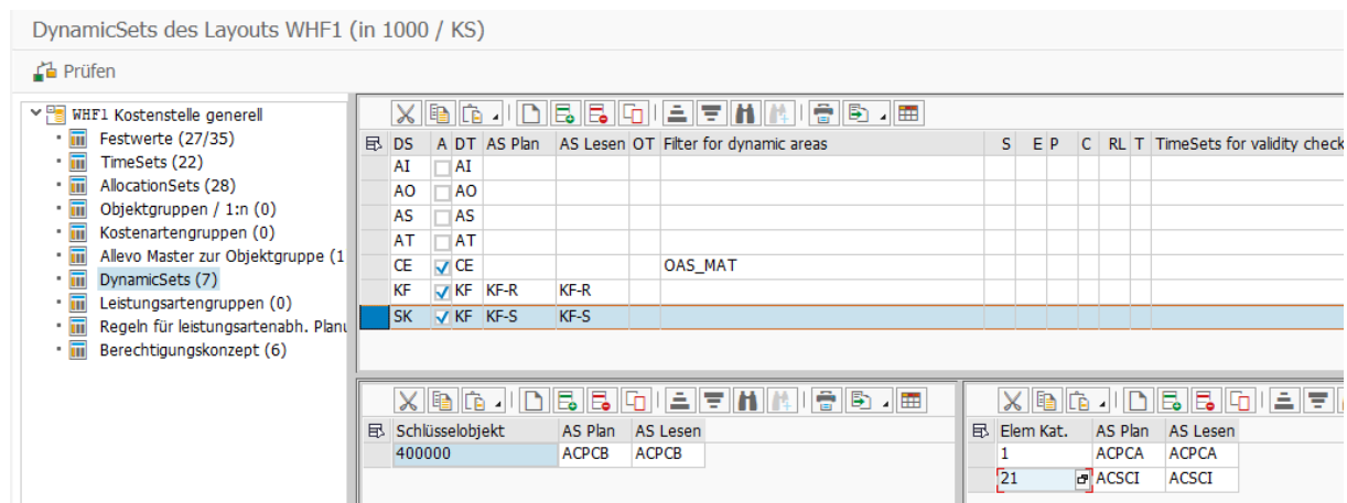
Abbildung 7-19: Einstellungen zu DynamikSets
