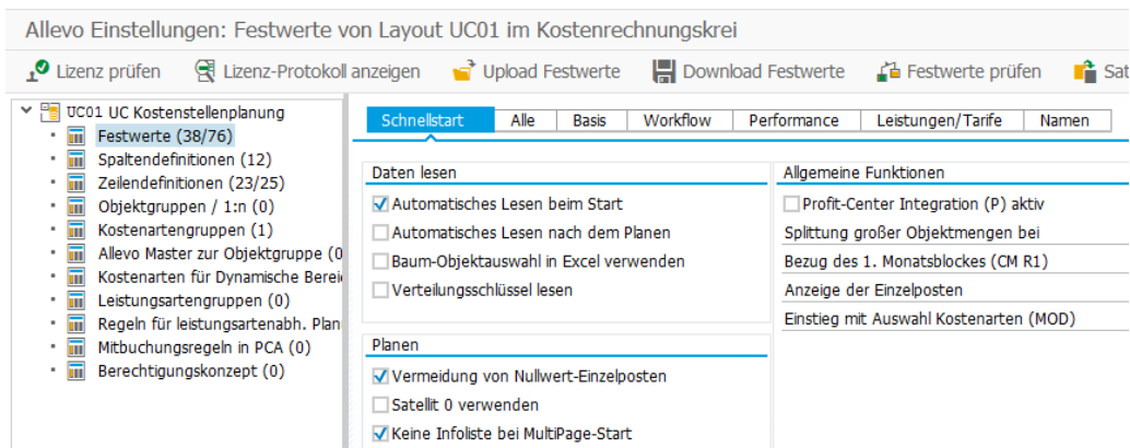
Abbildung 7-1: Übersicht der Einstellungen mit Navigationsbaum
