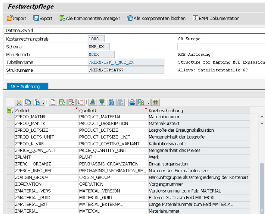
Abbildung 17-21: Feldzuordnung für Datenübernahme aus Materialkalkulation
