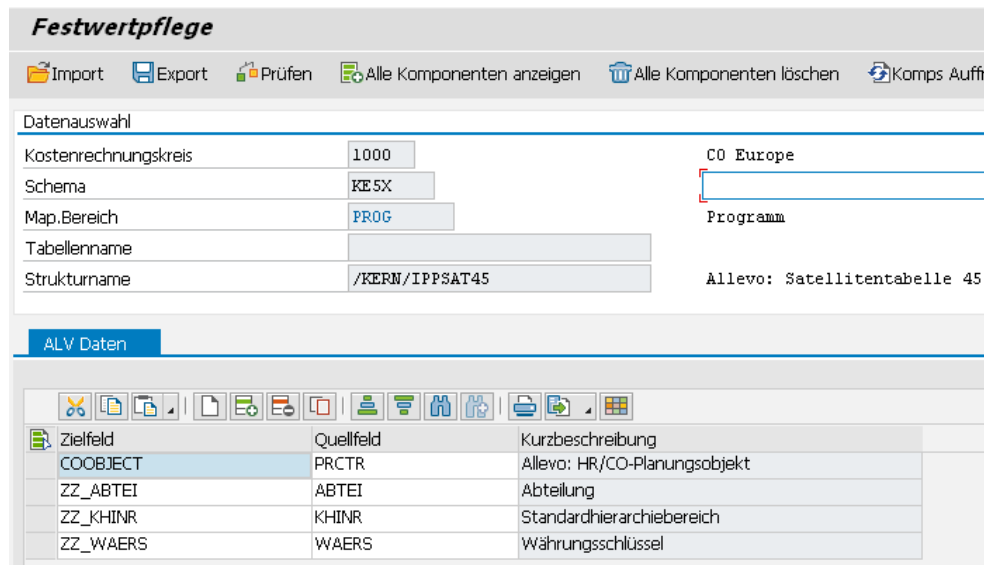
Abbildung 17-6: Feldzuordnung ALV Datenübernahme
