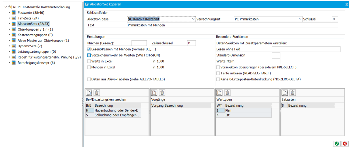
Abbildung 7-16: Eigenschaften zum AllocationSet
