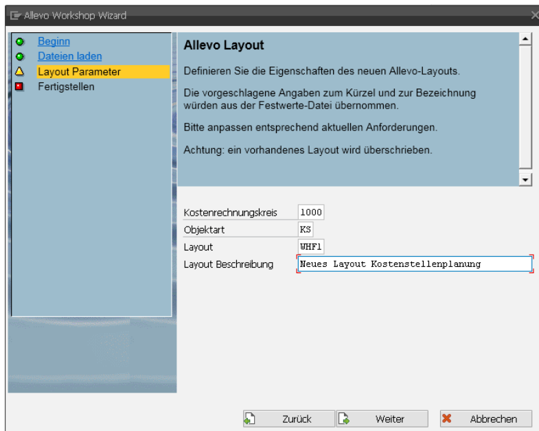
Abbildung 9-3: Allevo Wizard zur Anlage Allevo-Layout
