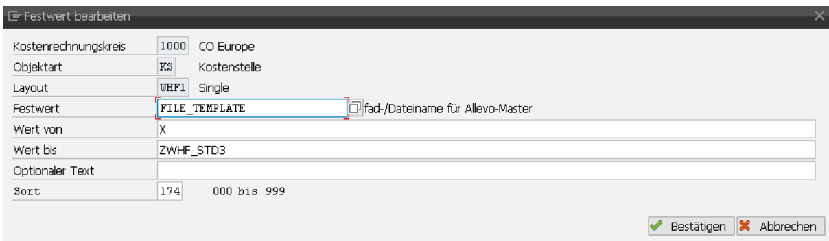
Abbildung 7-4: Allevo-Festwert bearbeiten
