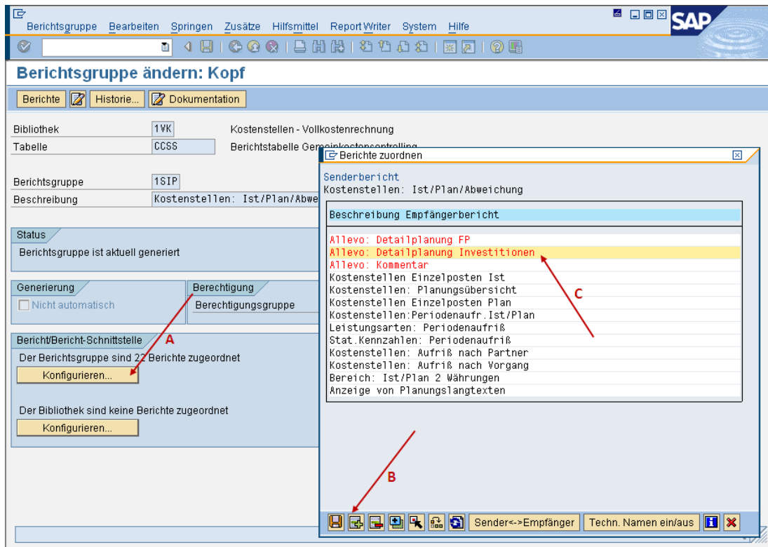
Abbildung 19-5: Einrichtung Bericht/Bericht-Schnittstelle
