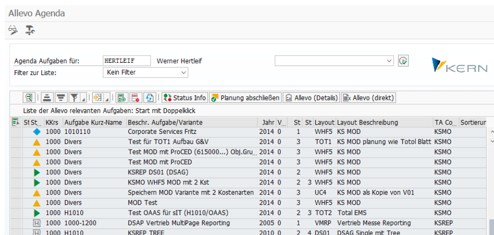
Abbildung 3-9: Allevo Planungs-Agenda
