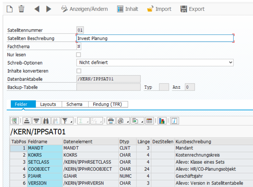
Abbildung 16-1: Satelliten-Details / Satelliten-Cockpit
